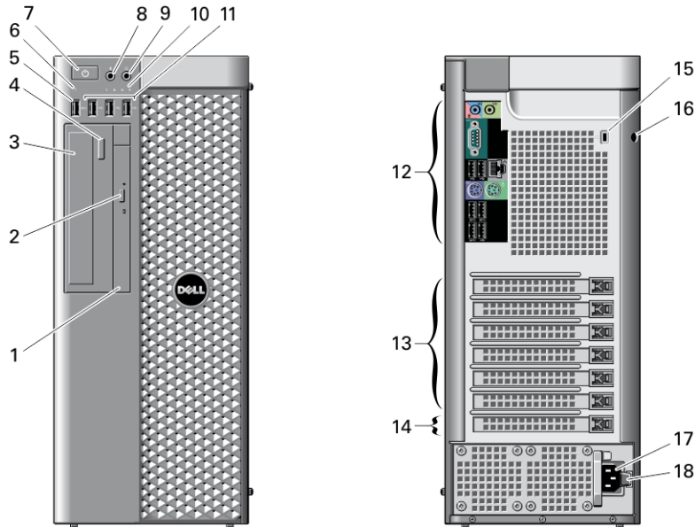
圖 1. T3610/T5610 的前視圖和後視圖
